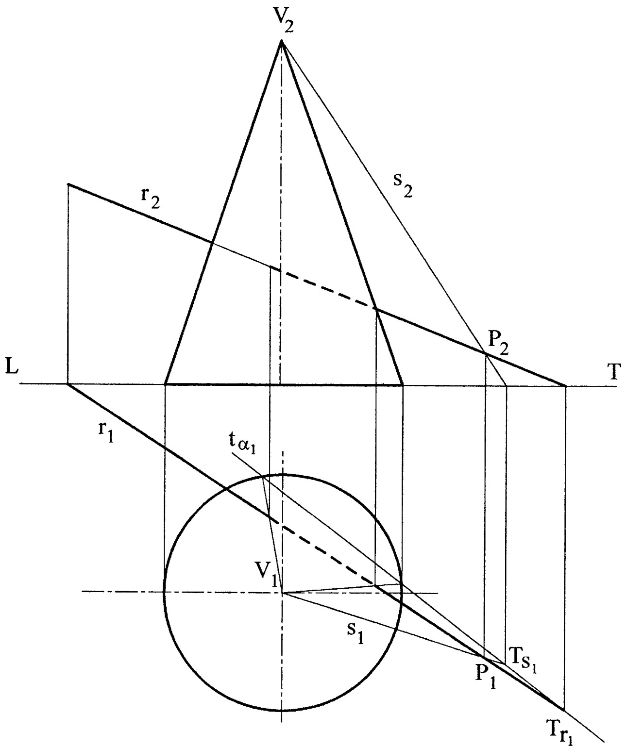
Punti di intersezione di una retta r con la superficie di un cono
