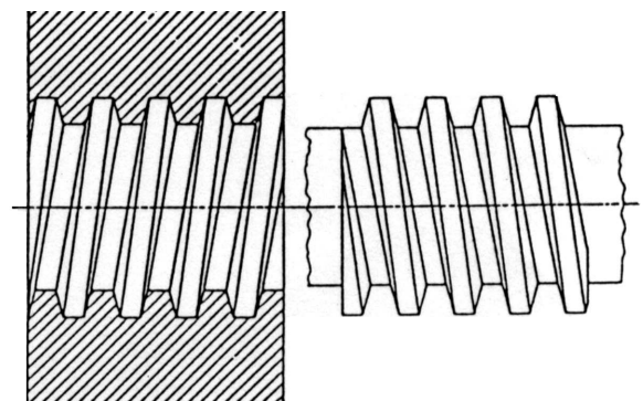
Coppia elicoidale
