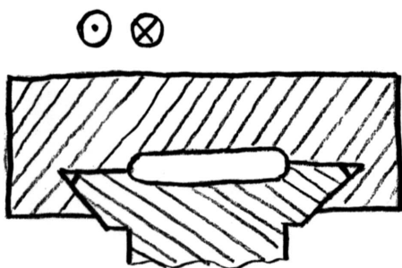
Coppia prismatica
