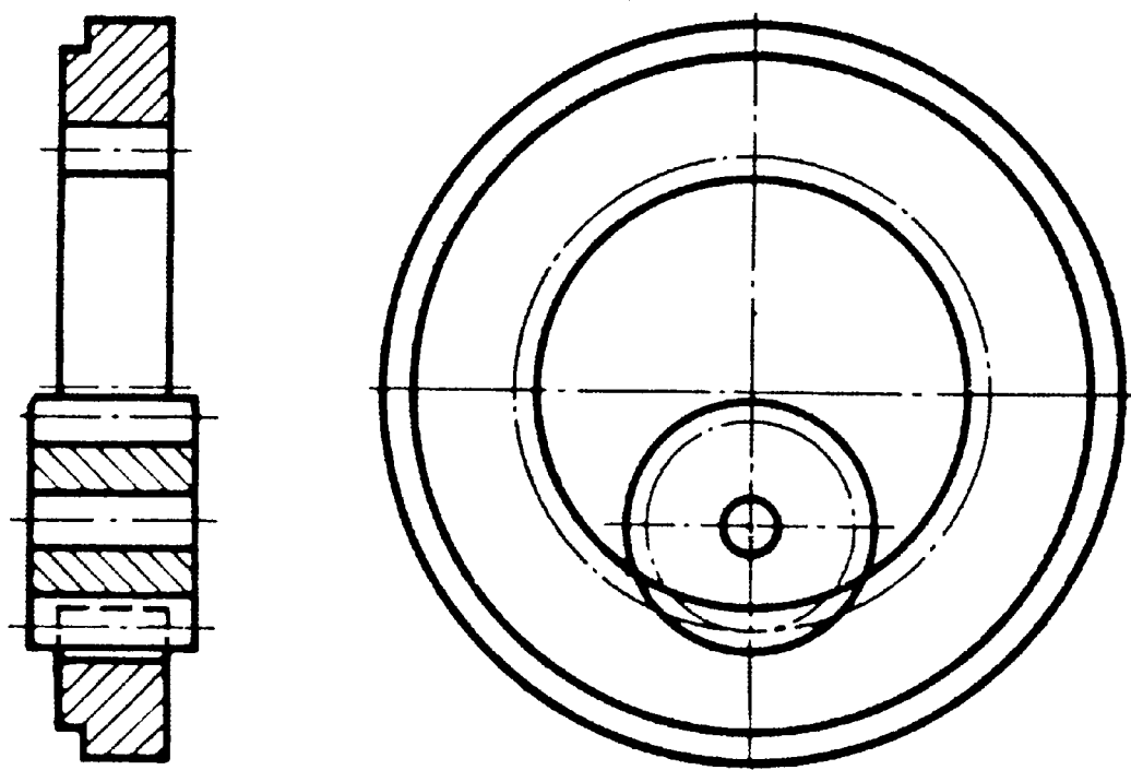
Rappresentazione convenzionale di un ingranaggio cilindrico interno
