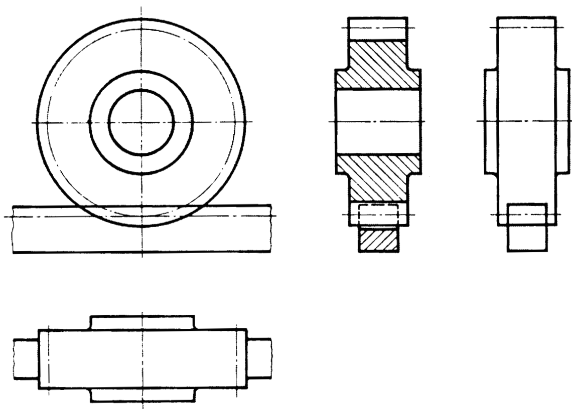
Rappresentazione convenzionale di un pignone con dentiera
